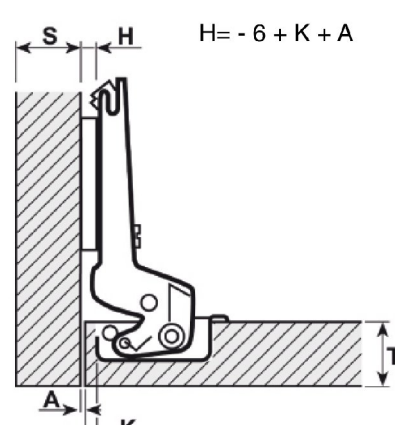
Applicazione con anta in luce Inset door installation
