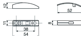
Lavorazione sull'anta per supporto ad incasso
