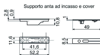
Supporto anta a ridosso e cover
